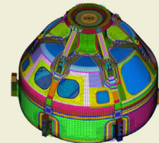
Composite Crew Module
