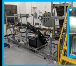
Lunar Auger Dryer ISRU (LADI)
