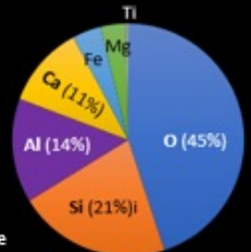
Legend: O, Si, Al, Ca, Fe, Mg, Ti
