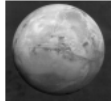
Image 1. Mars hemisphere.
